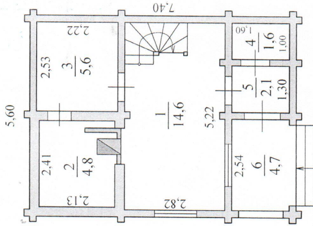
План этажа 1-й этаж М 1:100
