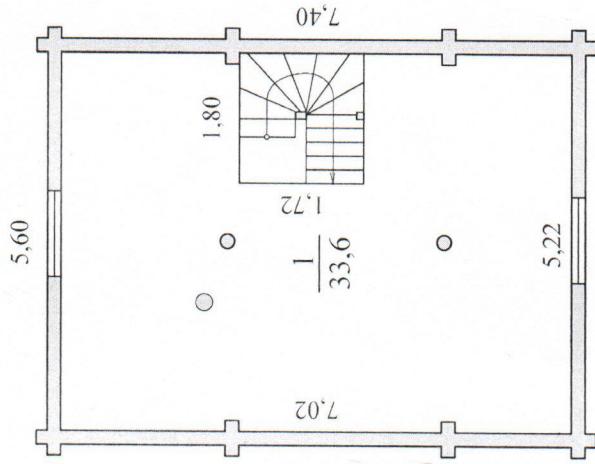
План этажа 2-й этаж (Мансардный) М 1:100
